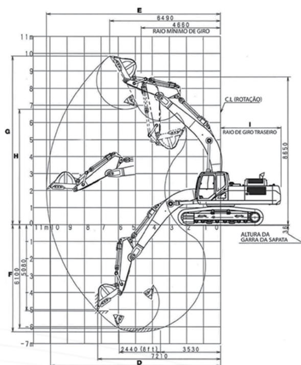
ALCANCE DE ESCAVAÇÃO COM BRAÇO DE 2,21 m
