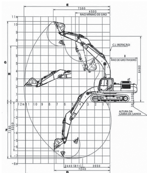
ALCANCE DE ESCAVAÇÃO COM BRAÇO DE 3,25 m
